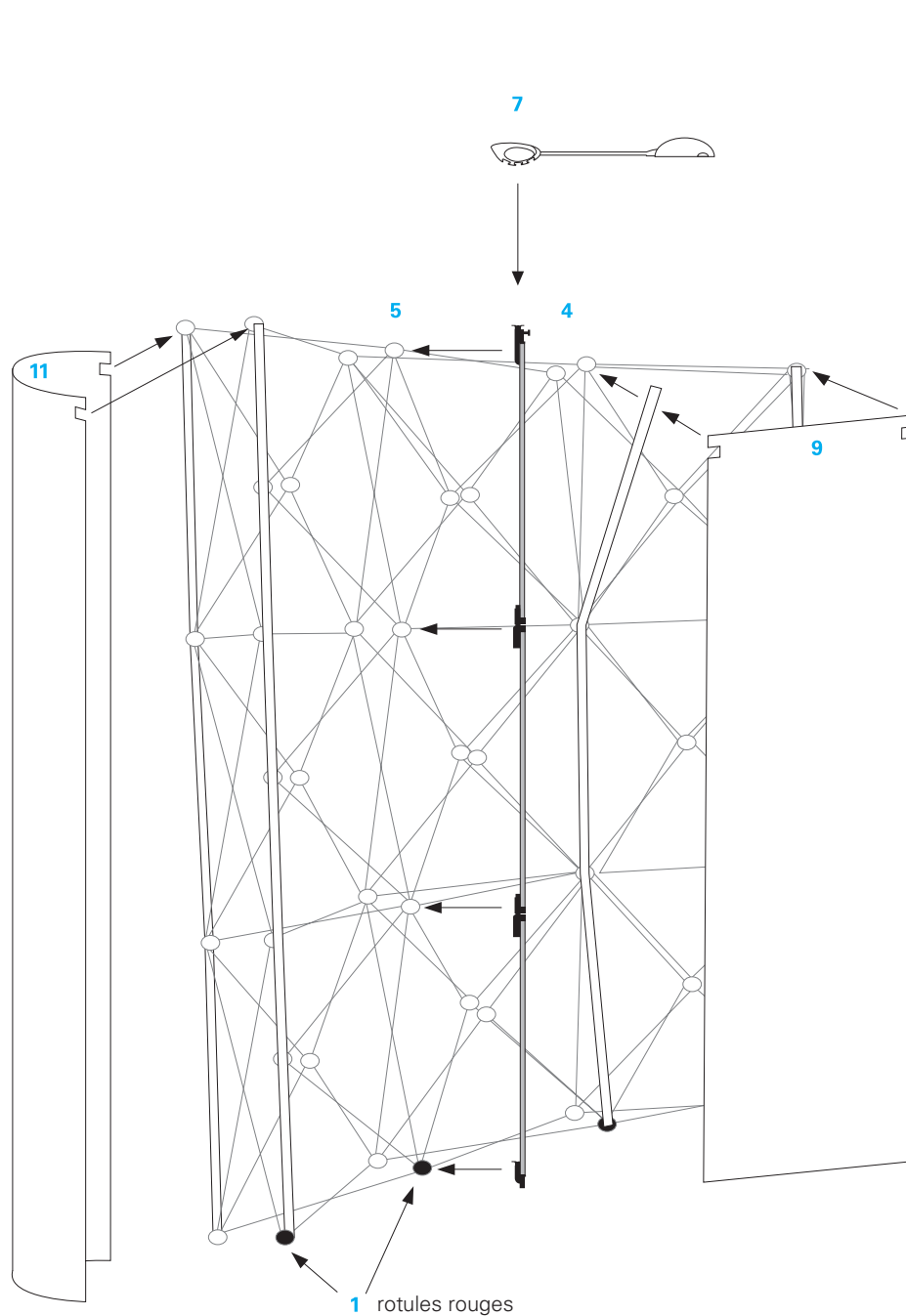
Exemple de configuration avec 3 lés de façade et 2 lés de retour.
